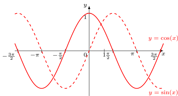
Graphes des fonctions sinus et cosinus
