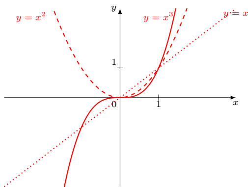
Graphes de fonctions puissances entières
