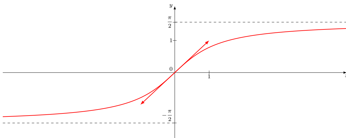
Graphe de la fonction arctangente
