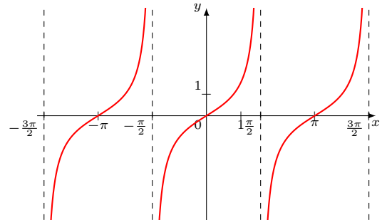
Graphes de la fonction tangente
