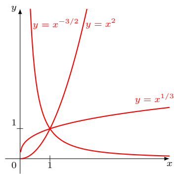
Graphes de fonctions puissances réelles
