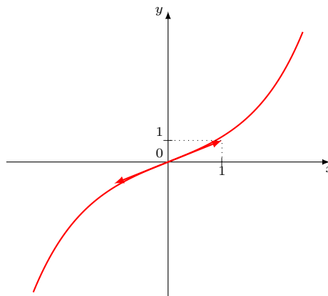
Graphe de la fonction sinus hyperbolique
