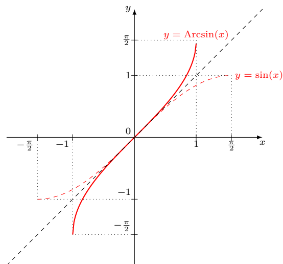
Graphe de la fonction arcsinus
