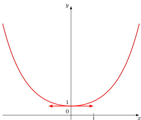
Graphe de la fonction cosinus hyperbolique
